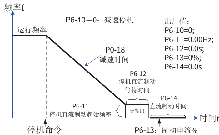
图 5-16 减速停车
