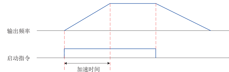
图 6-29 直接启动时序图
