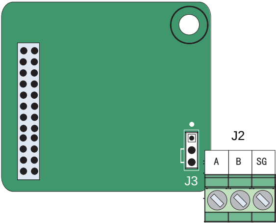
图 10-9 YD280E RS485 Card端子分布示意图
