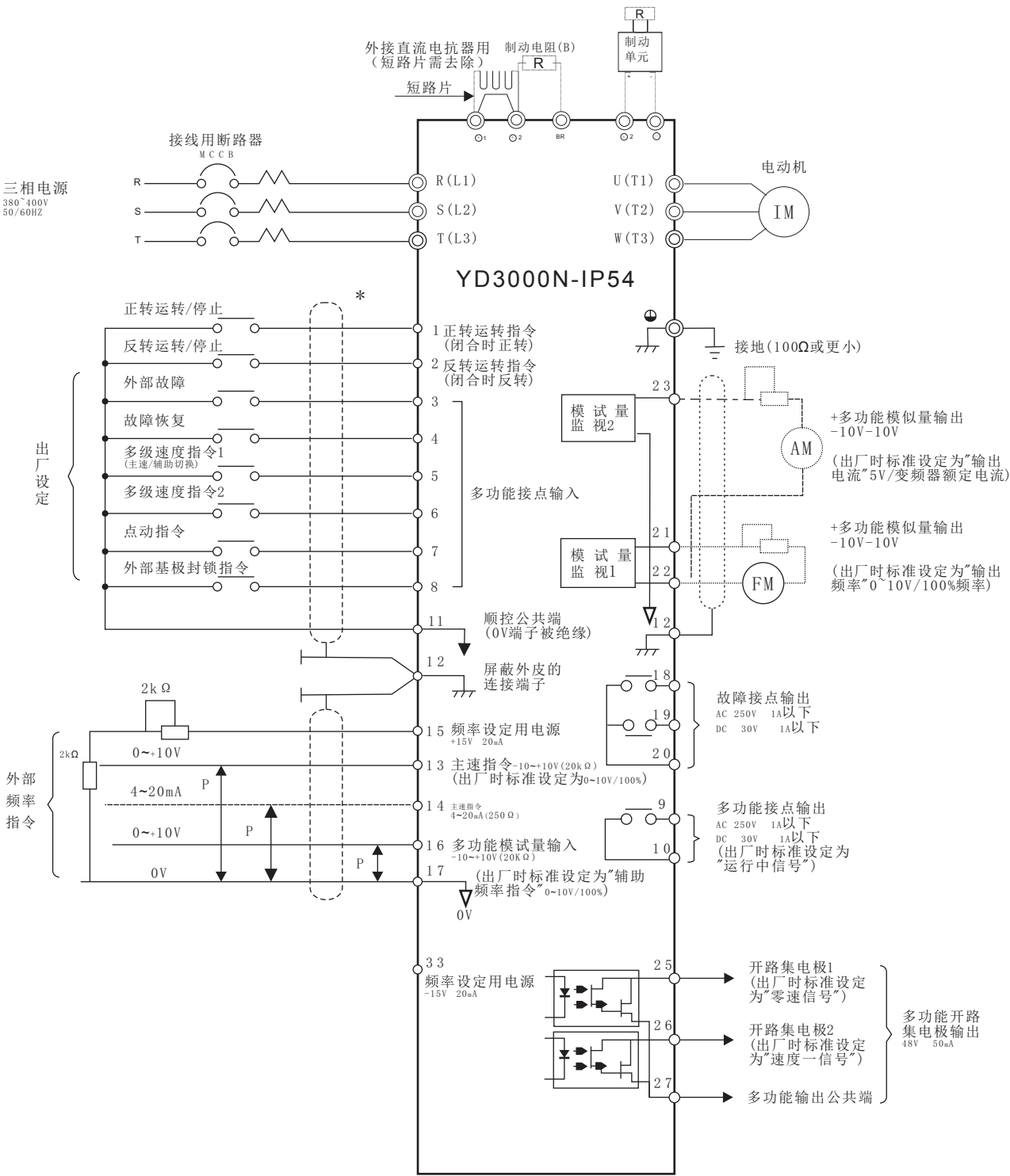
连接图 (以YD3185T4N-IP54 为例)
