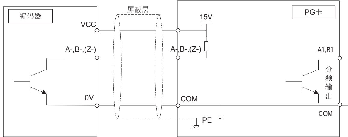
图 10-15 接口回路1
