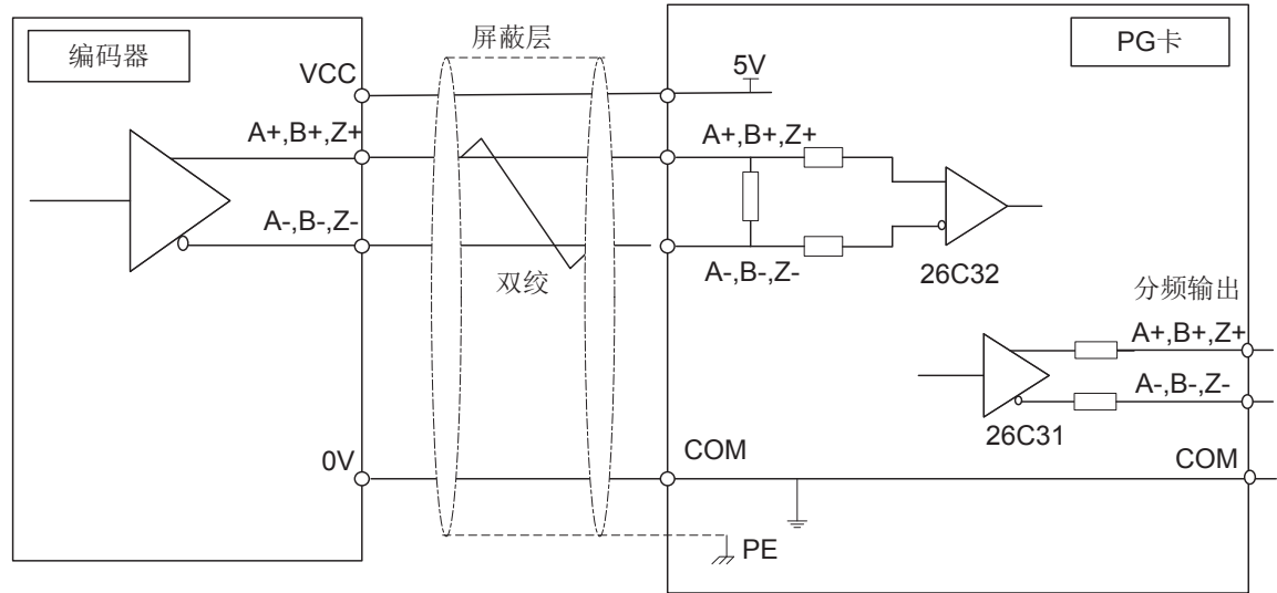
图 10-16 接口回路2
