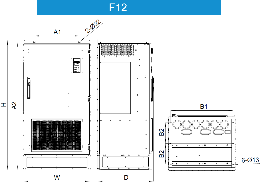
F12整机尺寸
