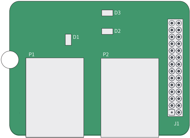
图 10-13 YD580-PN 卡端子分布示意图
