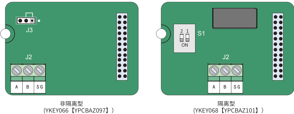
图 10-9 YD580-RS485 端子分布示意图
