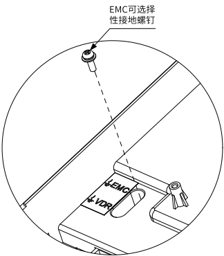
图3-69 断开EMC可选择性接地螺钉
