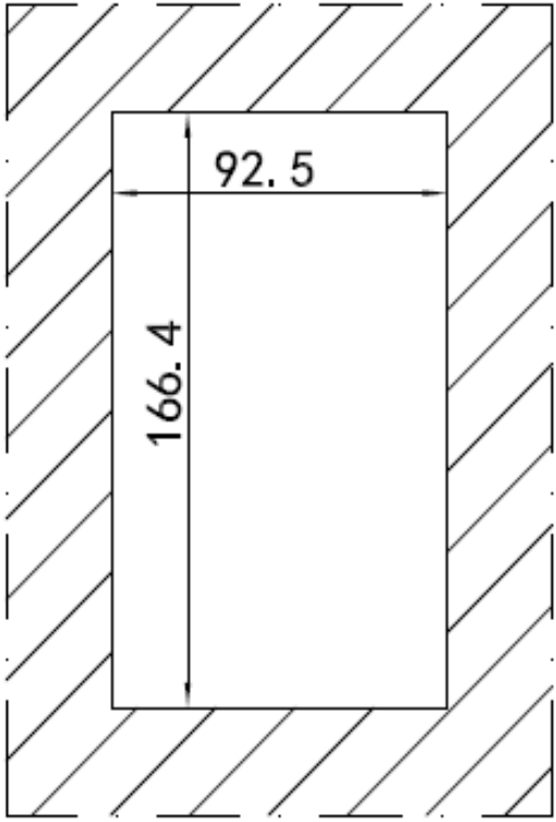
YD580-外引键盘仓开孔尺寸 (单位：mm)
