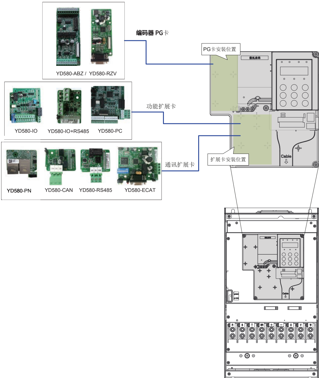
图 10-1 扩展卡的安装位置
