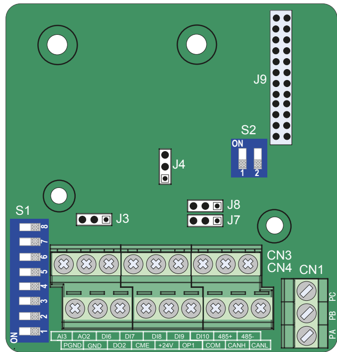
图 10-2 YD58IO1 端子分布示意图
