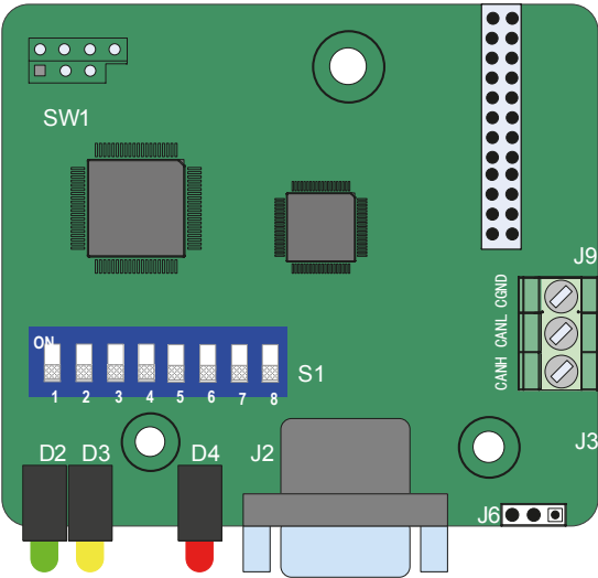
图 10-11 YD58DP2 端子分布示意图
