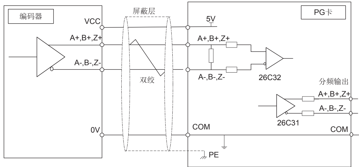
图 10-15 接口回路1
