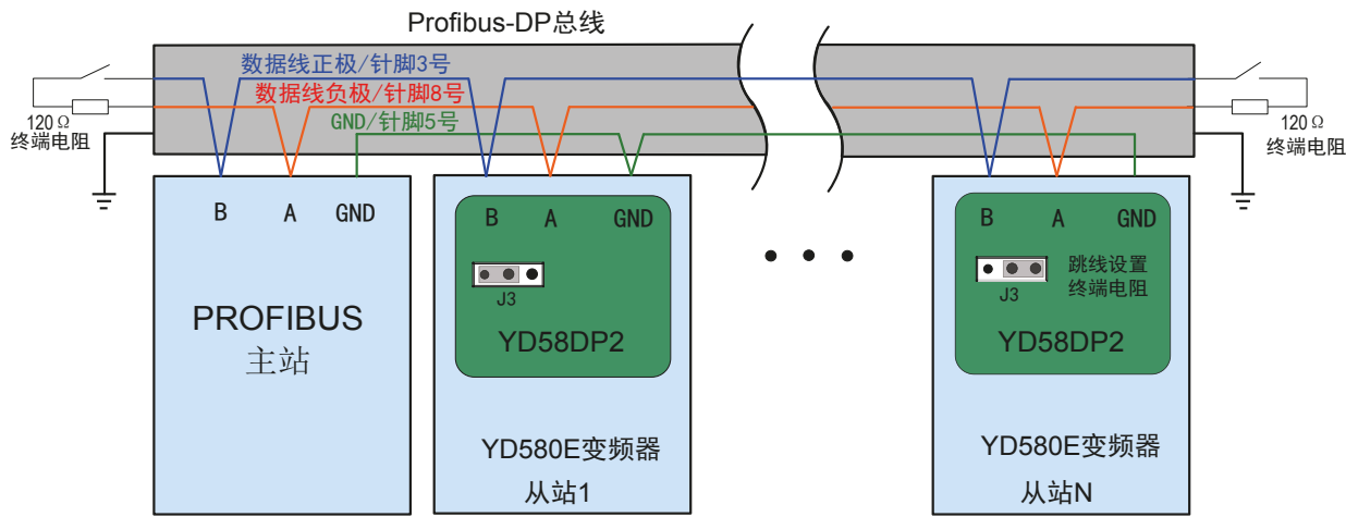
图 10-12 YD58DP2 卡与 Profibus 主站的连接示意图
