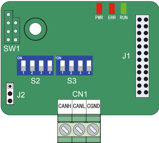
图 10-8 YD58CAN2 端子分布示意图
