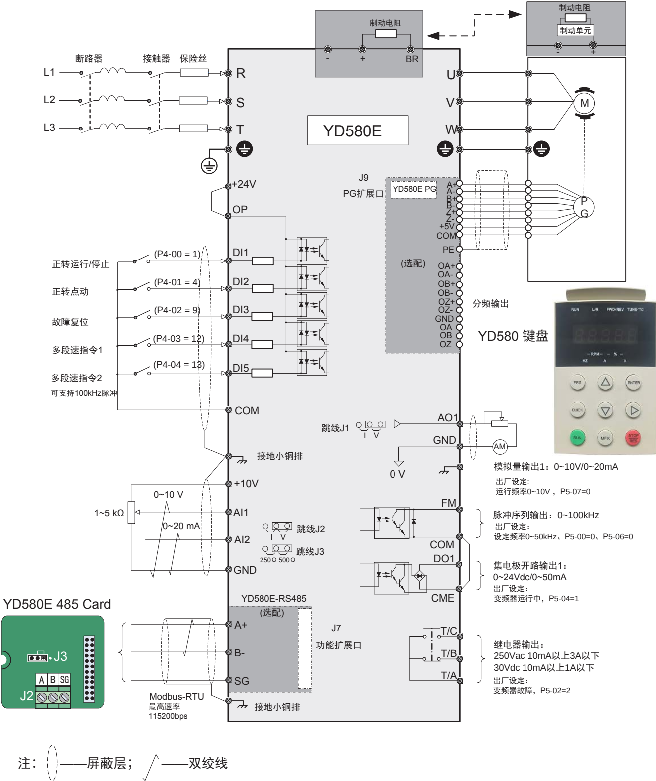
图 3-26 三相 380V~480V 典型接线图
