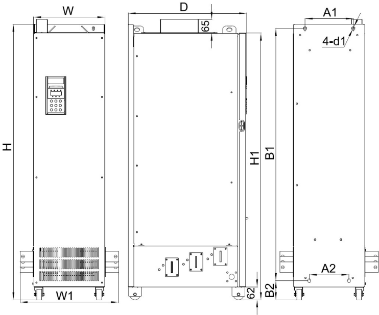
图 9-4 YD580ET4-200G/220P~YD580ET4-450G/500P 外型尺寸及安装尺寸示意图
