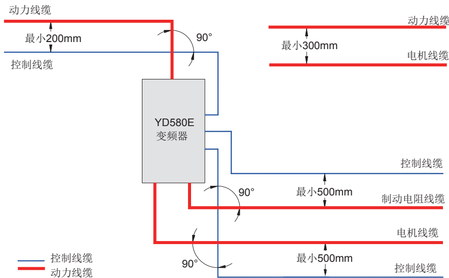
图 3-59 电缆布线图
