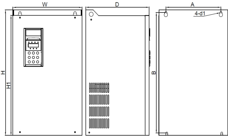
图 9-2 YD580ET4-30G/37P(B)-T~YD580ET4-160G/200P-T 外型尺寸及安装尺寸示意图
