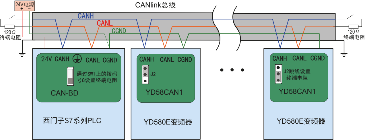
图 11-7 CANlink 总线连接拓扑结构
