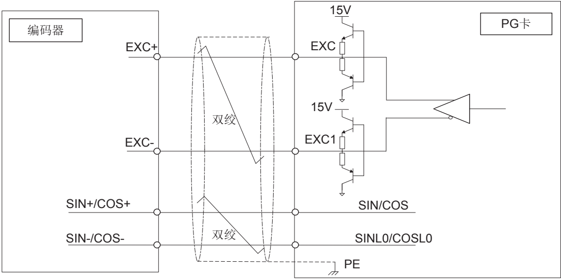
图 10-14 YD580-RZV 接口回路
