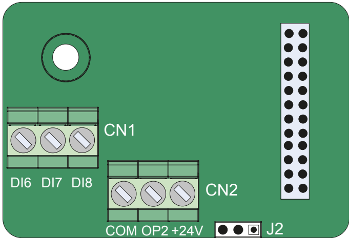
图 10-3 YD58IO2 端子分布示意图
