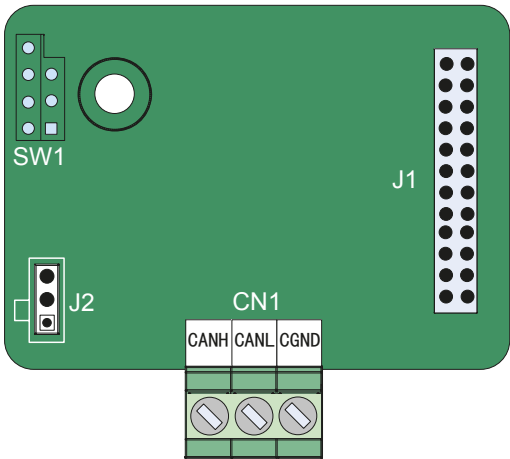
图 10-6 YD58CAN1 端子分布示意图
