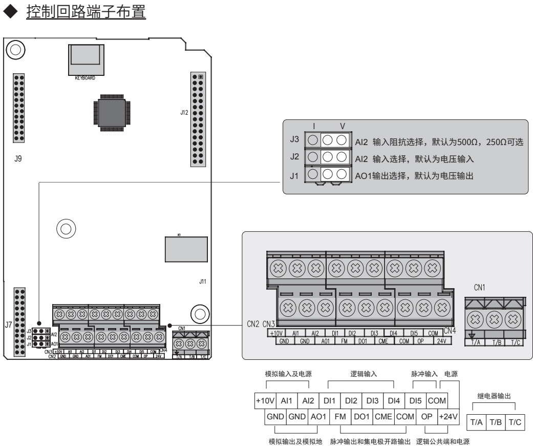
图 3-57 控制回路端子布置图
