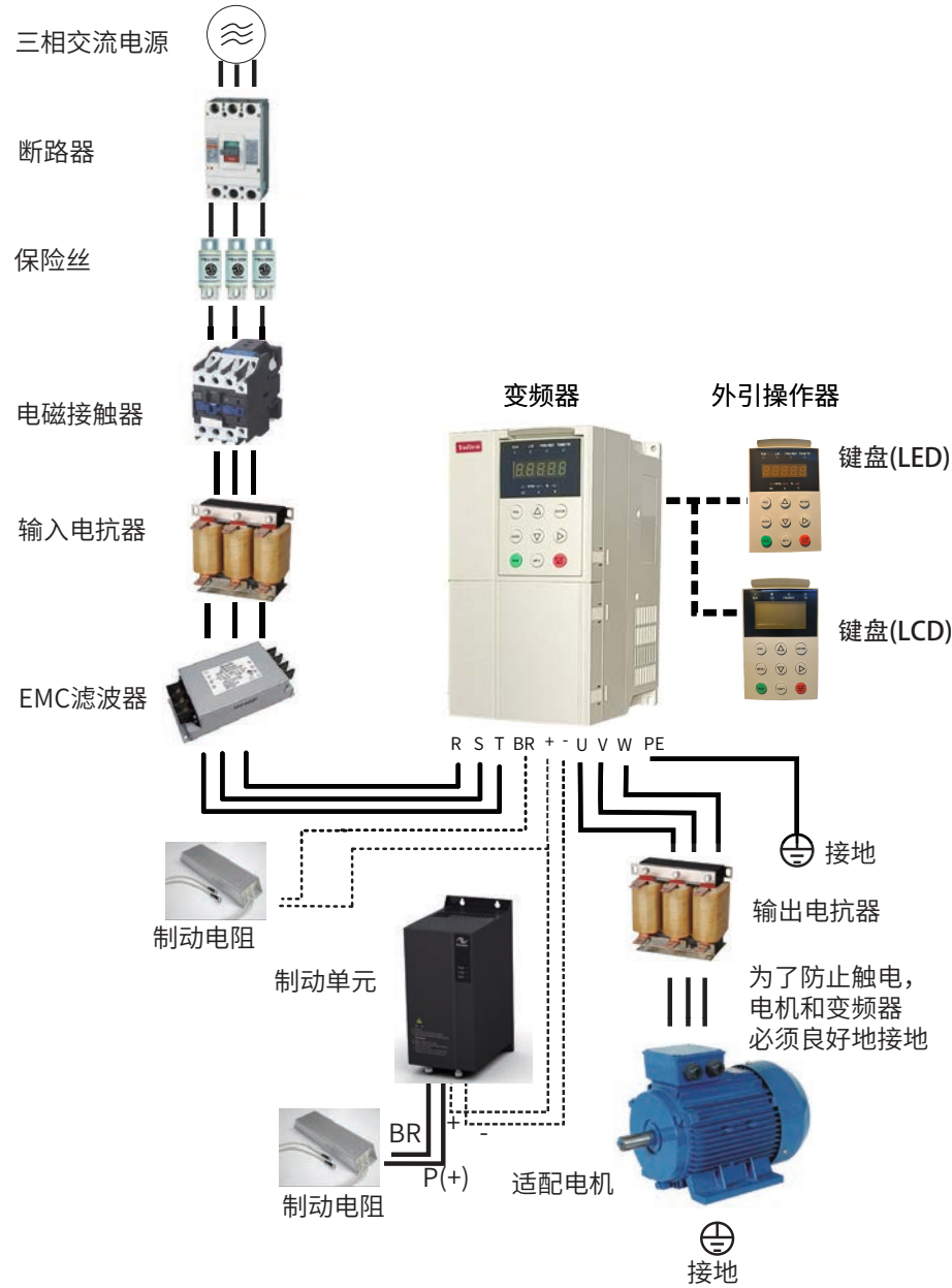
图 2-1 YD580E 系列系统构成
