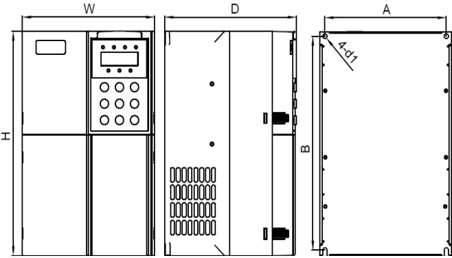
图 9-1 YD580ET4-0P7G/1P5PB ~ YD580ET4-22G/30PB 外型尺寸及安装尺寸示意图
