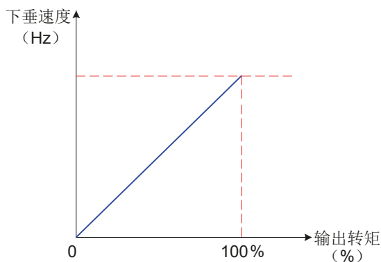
图 6-54 下垂速度与输出转矩关系示意下垂速
